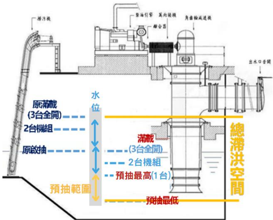
圖一 抽水站預抽與強化預抽示意圖
